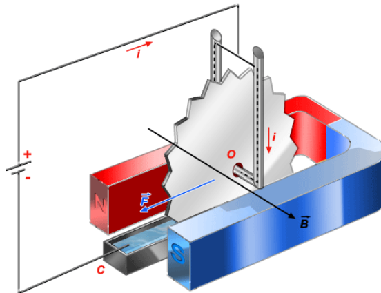
Figura 30. A roda de Barlow.
