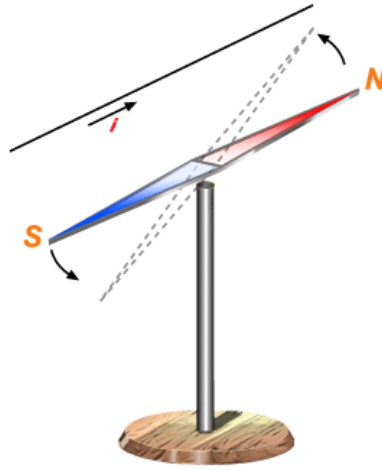
Figura 18. A experiência de Oersted.
