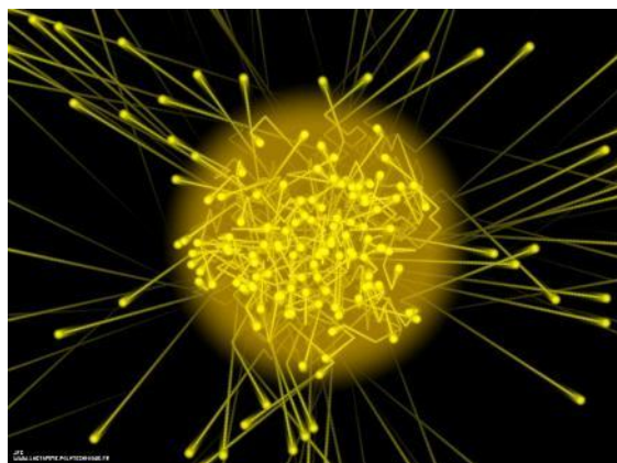
Figura 39. Luz é composta por fótons.
