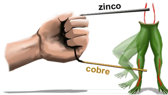
Figura 16. Esquema do experimento de Luis Galvani.
