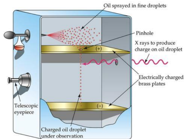
Figura 38. A experiência de Millikan
