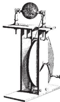
Figura 11. A primeira máquina elétrica, construída por Hauksbee.
