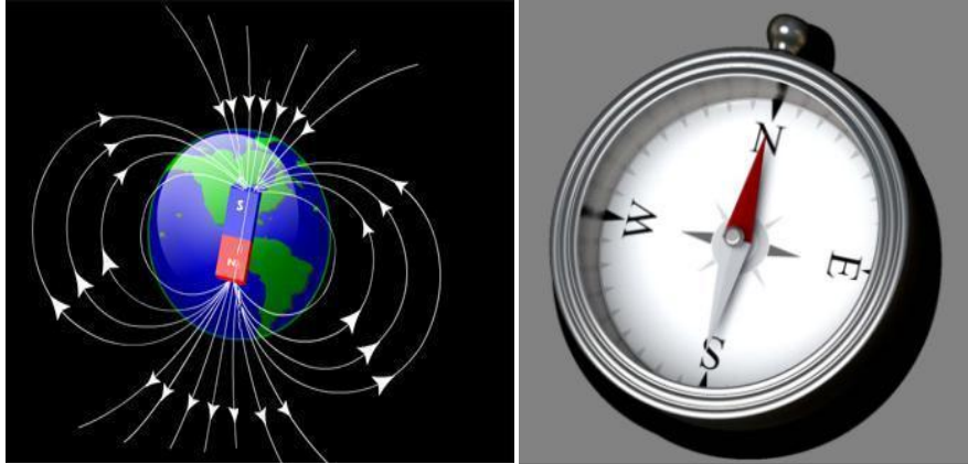
Figura 5. A bússula funciona por conta da existência do campo magnético da Terra.
