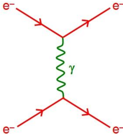
Figura 42. Fótons são partículas intermediárias das interações eletromagnéticas.
