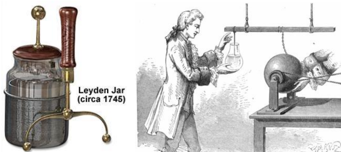
Figura 13. A garrafa de Leyden.
