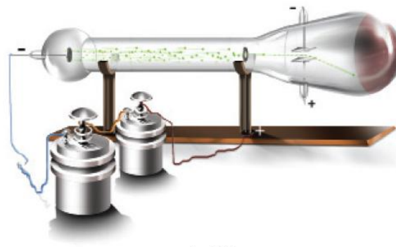
Figura 37. Arranjo para produzir Raios catódicos e defletí-los.
