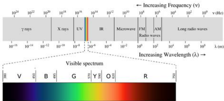
Figura 34. O espectro eletromagnético.
