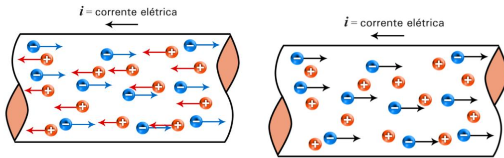
Figura 24. Concepção de Ampère sobre a corrente elétrica e a concepção atual. Utilizava, na sua teoria, as palavras eletricidade positiva e negativa.
