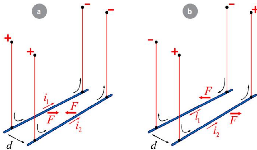
Figura 21. A experiência de Ampère.
