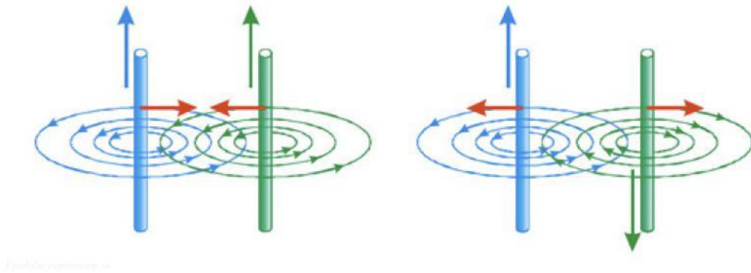
Figura 22. Cada fio gera um campo magnético que influencia o outro.
