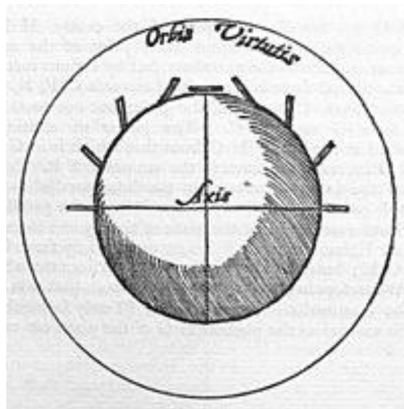
Figura 9. O conceito de Orbis Virtutis e as linhas de campo.
