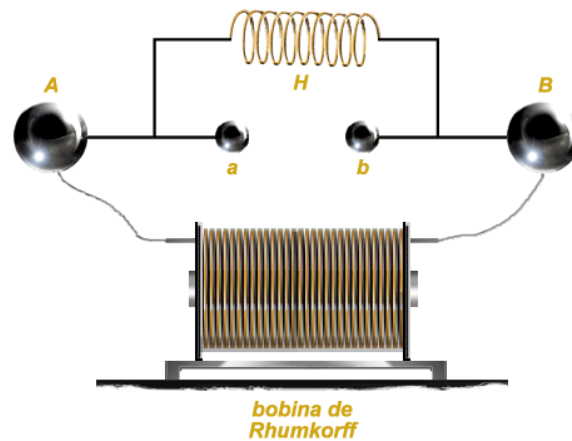
Figura 36. Arranjo experimental de Hertz.
