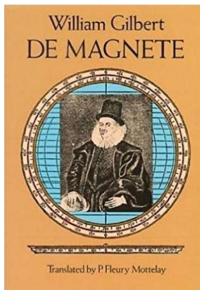
Figura 8. William Gilbert e seu versorium .
