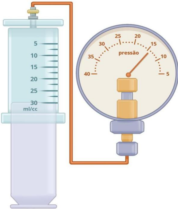
Fig. 1- Manômetro.
