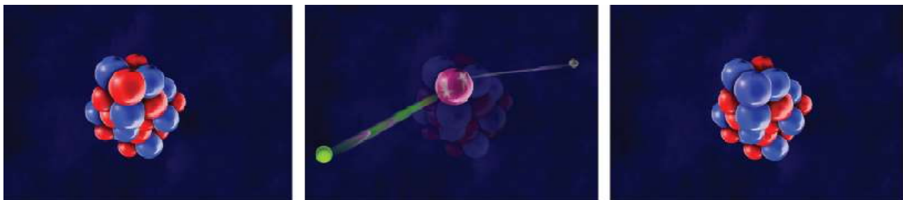
Fig. 6- Transmutação de um elemento químico.
