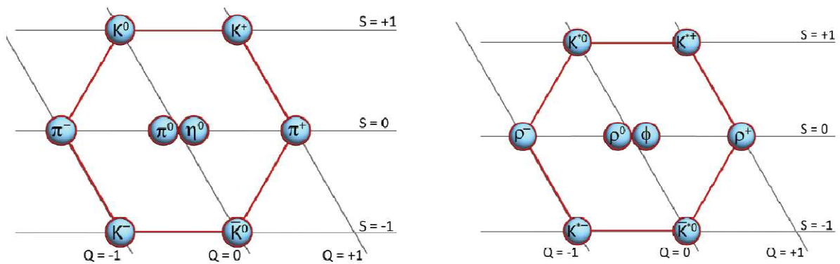
Fig. 8- Os oito mésons escalares e os mésons vetoriais.
