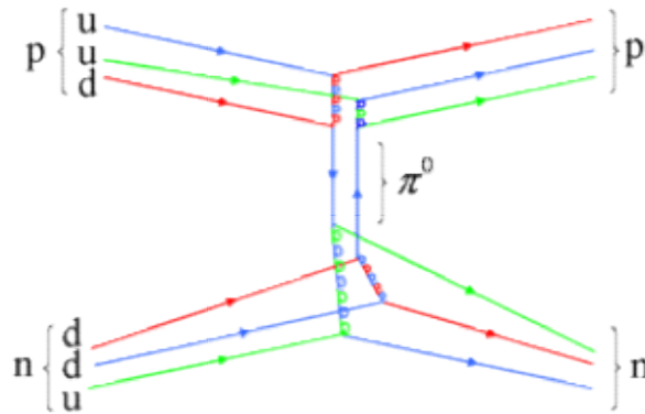
Fig. 3- O mesmo diagrama com o quark individual constituinte.
