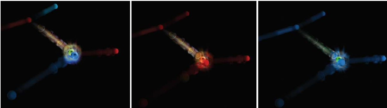
Fig. 1- Na teoria de Yukawa a partícula trocada, ou intermediária, seria o méson \pi .
