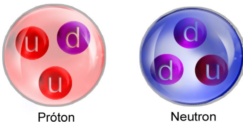
Fig. 11- Prótons e nêutrons são constituídos a partir de três quarks.
