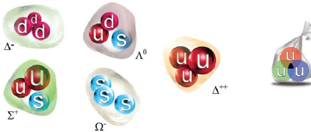
Fig. 9- Bárions são partículas constituídas a partir de três quarks.
