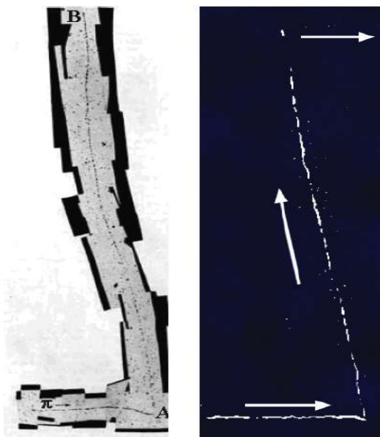
Fig. 2- Uma das emulsões fotográficas que fizeram história.
