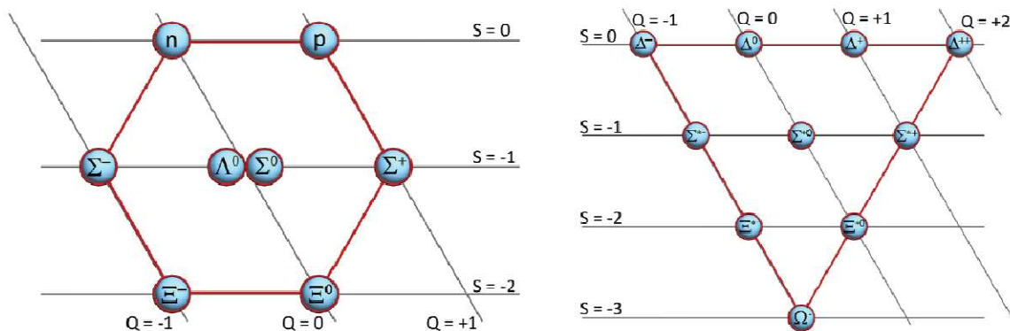
Fig. 10- Alguns bárions e suas relações com simetrias.
