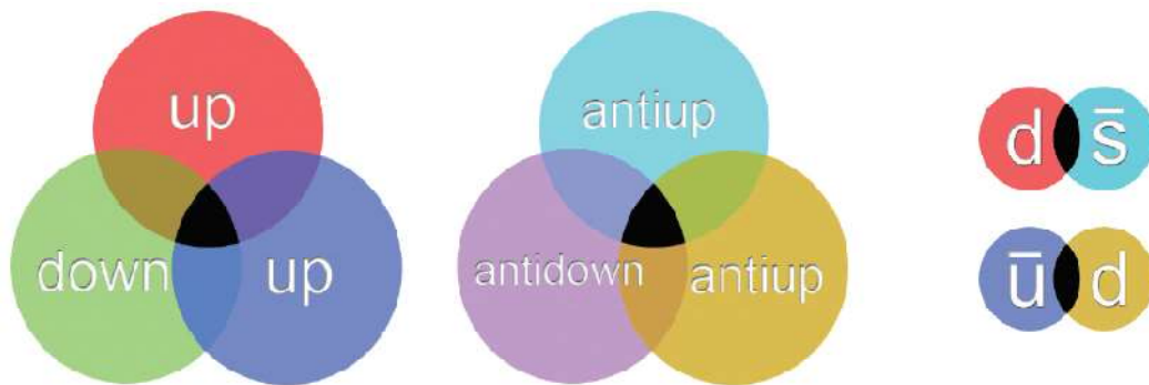
Fig. 13- Bárions e mésons são constituídos de quarks com cores distintas ou anticores distintas. Mésons são constituídos de quarks de uma cor e antiquarks, da cor oposta. Os objetos formados são destituídos de cor.
